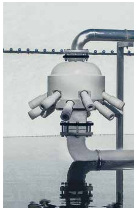
12 路射流曝气器, 材质 PP
