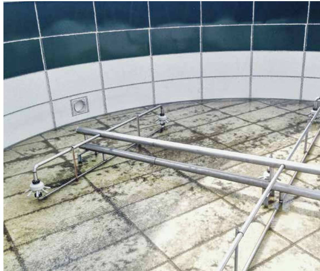
在 2200m 3 曝气池内安装的7路射流器, 位于巴西, 食用油生产工业
