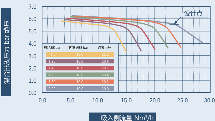
液体喷射气体压缩机的特性曲线
