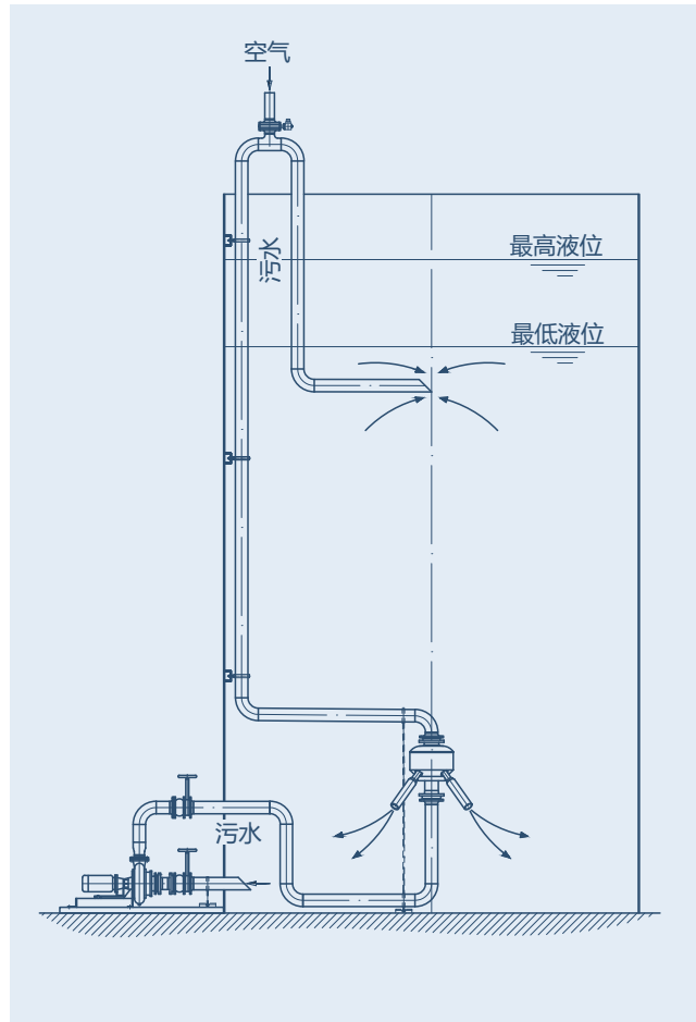
空气 SBR 系统
